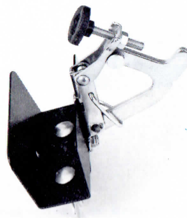
Felgenspanner in geöffneter Stellung
